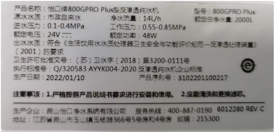
800GPRO Plus (铭牌)
